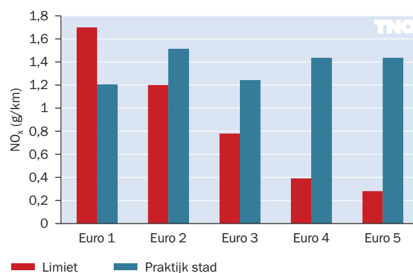
Figuur 3. \text{NO}_x -emissies van zware bestelwagens in de stad, in vergelijking met de emissielimiet.
